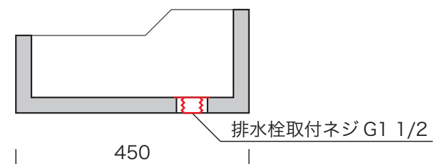
断面
